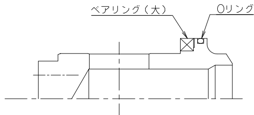
シャフト
